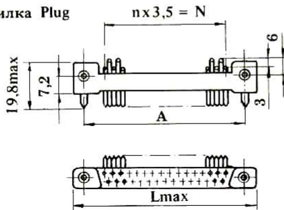
Вилка Plug
